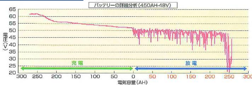
バッテリーデータロガー
